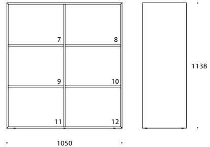
Art.nr 4660-2 Skåp 2 Cabinet 2
